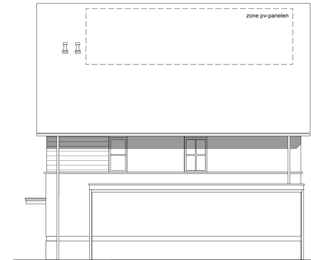
Zijgevel rechts bwnr 61
